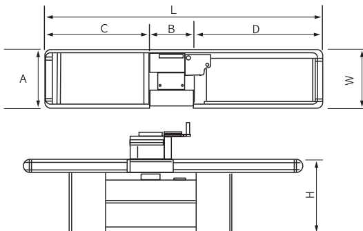
● 신형알루미늄컨베이어계산대(무동력)
