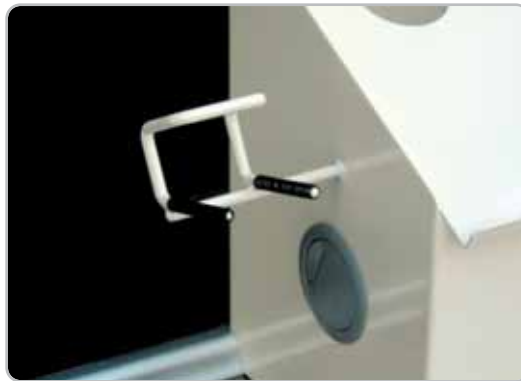
● 핸드스캐너 걸이대 WS-015-03 고무를 코팅하여 스캐너에 흠집이 생기지 않도록 보호합니다.
