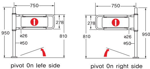
● 스윙게이트 WS-026-02 1600W x 950H X 1000D
